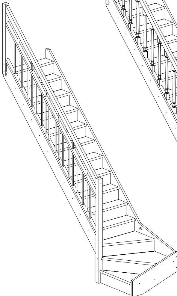
mit Designgeländer
