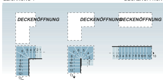
ZEICHNUNG 4
