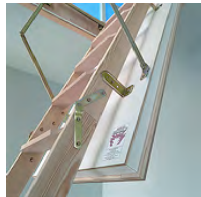
Detailansicht
