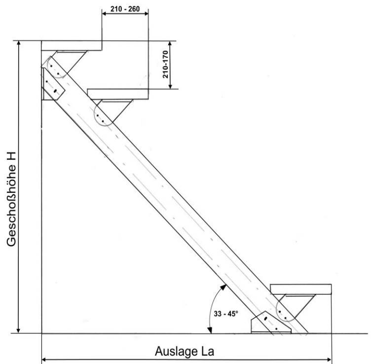
Verstellbereich MonoBeam Einholmtreppe
